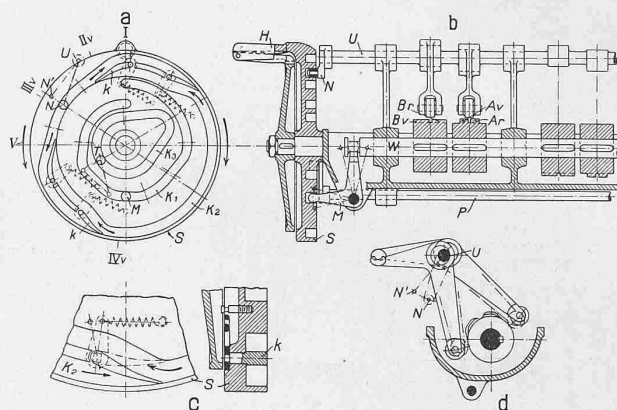
Abb. 7 a bis d. Schema der Umsteuerung
