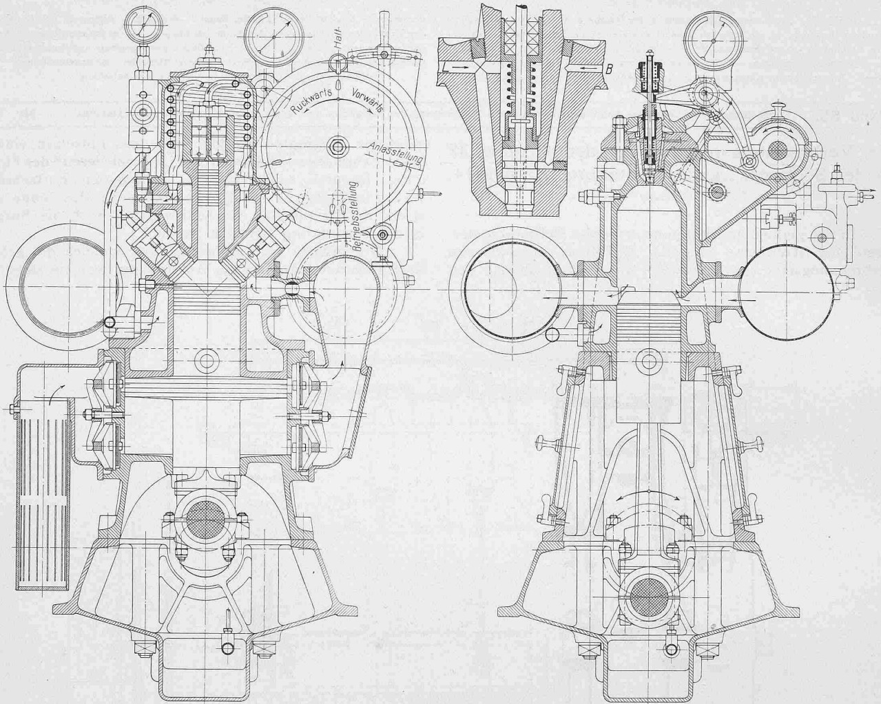
Abb. 5. Umsteuerbarer Zweitakt-Schiffs-Dieselmotor der Schweiz. Lokomotiv- und Maschinenfabrik Winterthur für 40 PS bei 500 Uml/min. Kompressor- und Zylinder-Querschnitte. — Masstab 1:10 (Detail vom Anlass- und Brennstoff-Ventil 1:3).
