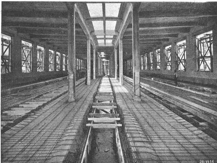
Tramremise der städtischen Strassenbahn Zürich
