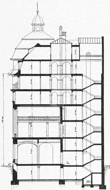
Abb. 7. Schnitt. — Masstab 1:400.
