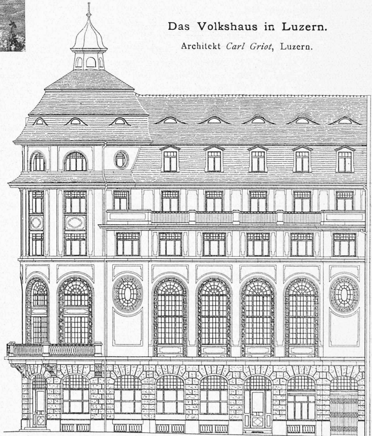
Abb. 8. Fassade an der Pilatusstrasse. — Masstab 1:250.
