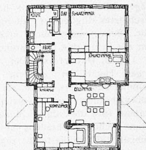
Ansicht von Südwest. — Grundrisse 1:500.
