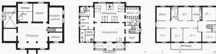
Grundrisse. — Masstab 1:500.
