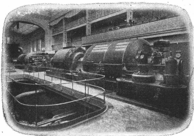
10 000 PS-Turbogenerator-Gruppen im Elektrizitätswerk der Stadt Stockholm.
