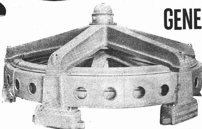
Drehstromgenerator 500 KVA, 7000—7500 Volt, 50 Cycles, 40 Touren, für Bremen.
