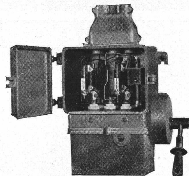
Automatische Schaltkasten mit Maximal-Strom- und Minimal-Spannungs-Auslösung.
