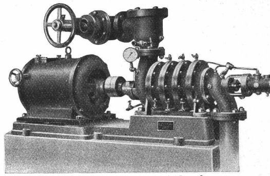
Vierstufige Hochdruckzentrifugalpumpe
