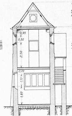
Abb. 2. Transformatoren-Häuschen Zuoz. — 1 : 200.
