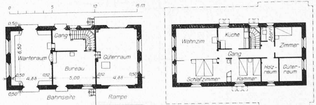
Abb. 3. Typus der Zwischen-Stationen. Grundrisse 1 : 400.
