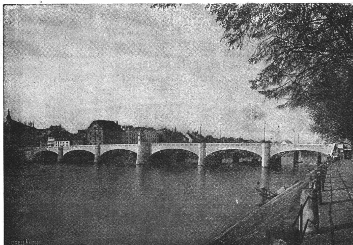
Mittlere Rheinbrücke in Basel, 200 m lang u. 18 m breit (Verkleidung sämtlicher Flächen in Götthardgranit).
