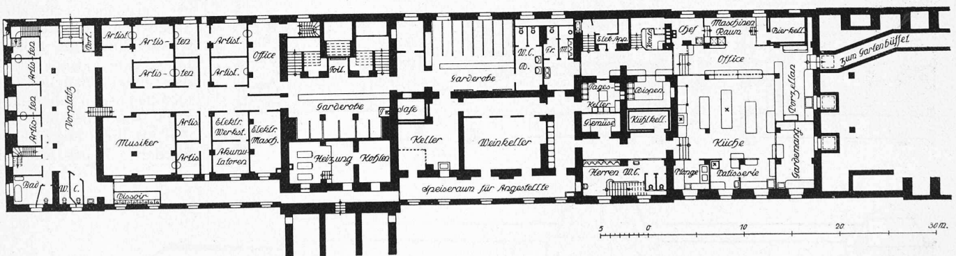
Abb. 7. Grundriss vom Untergeschoss. — Masstab 1 : 500.
