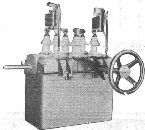
Ölschalter mit direkter Maximalauslösung
