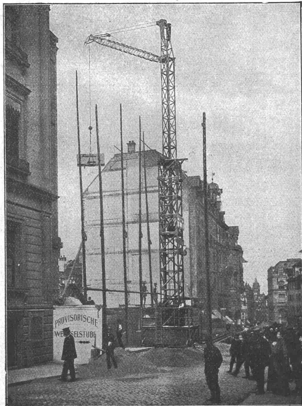
1 fahrbarer Turmdrehkran mit einem Motor ohne Wendegetriebe für Heben und Fahren. Zwei Hubgeschwindigkeiten, 1,5–3 t Tragkraft, 9–5 m Aus- ladung, 19–26 m Rollenhöhe. Veränderliche Ausladung. Kran an der Handelsbank Basel.
