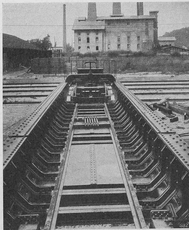
Abb. 4. Blick auf die Fahrbahn der Ladebrücke.
