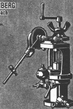
Schmierapparat
