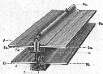
b) Duplexsprosse.
