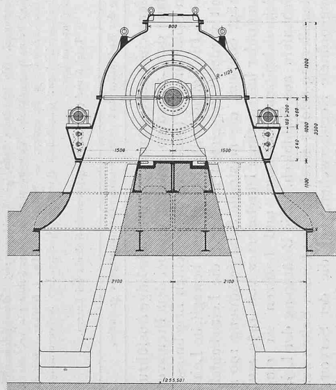
Abb. 14. Schnitt durch ein Wellenlager mit Bedienungskessel. — 1 : 75.
