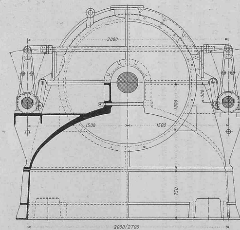
Abb. 13. Mittel-Querschnitt durch Welle und Doppelsaugkessel. — 1 : 50.
