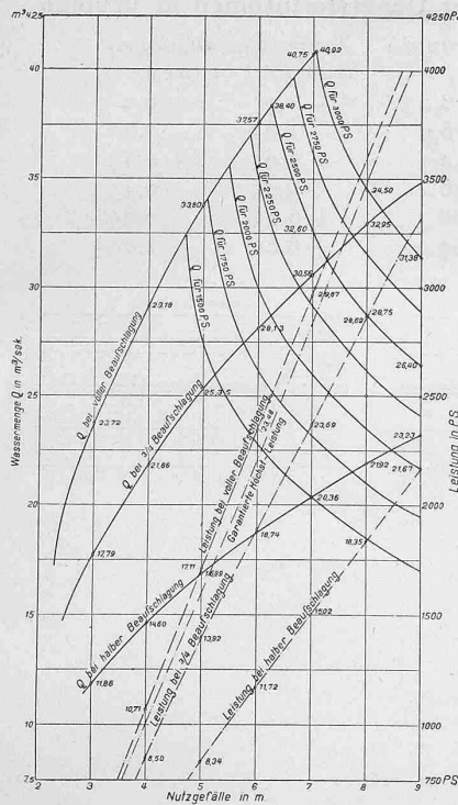
Abb. 17. Wassermenge- und Leistungskurven berechnet auf Grund der Laufrad-Bremssversuche in Abb. 16 (Seite 16).
