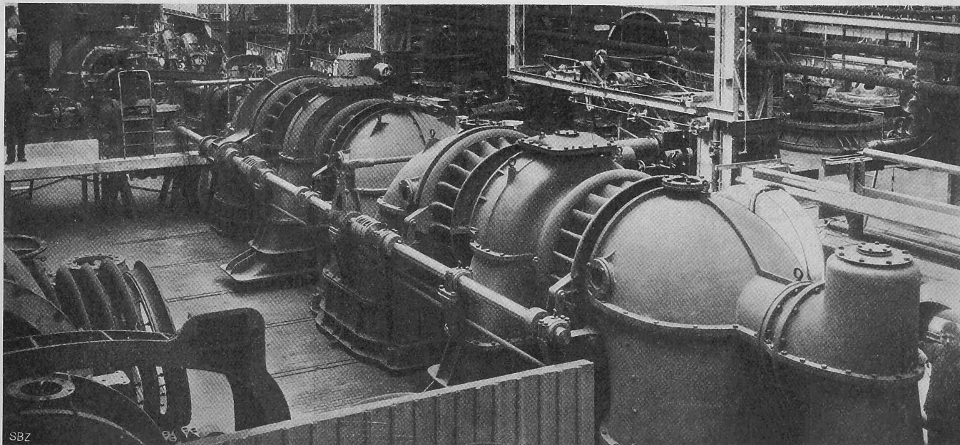
Abb. 15. Vierfache Francis-Turbine für normal 2200 PS, gebaut von J. M. Voith in Heidenheim a. d. Brenz.
