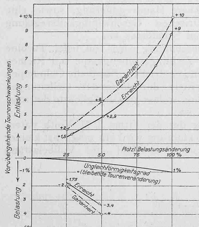
Abb. 22. Uebersicht der Garantie- und Versuchszahlen der Geschwindigkeits-Regulierung.
