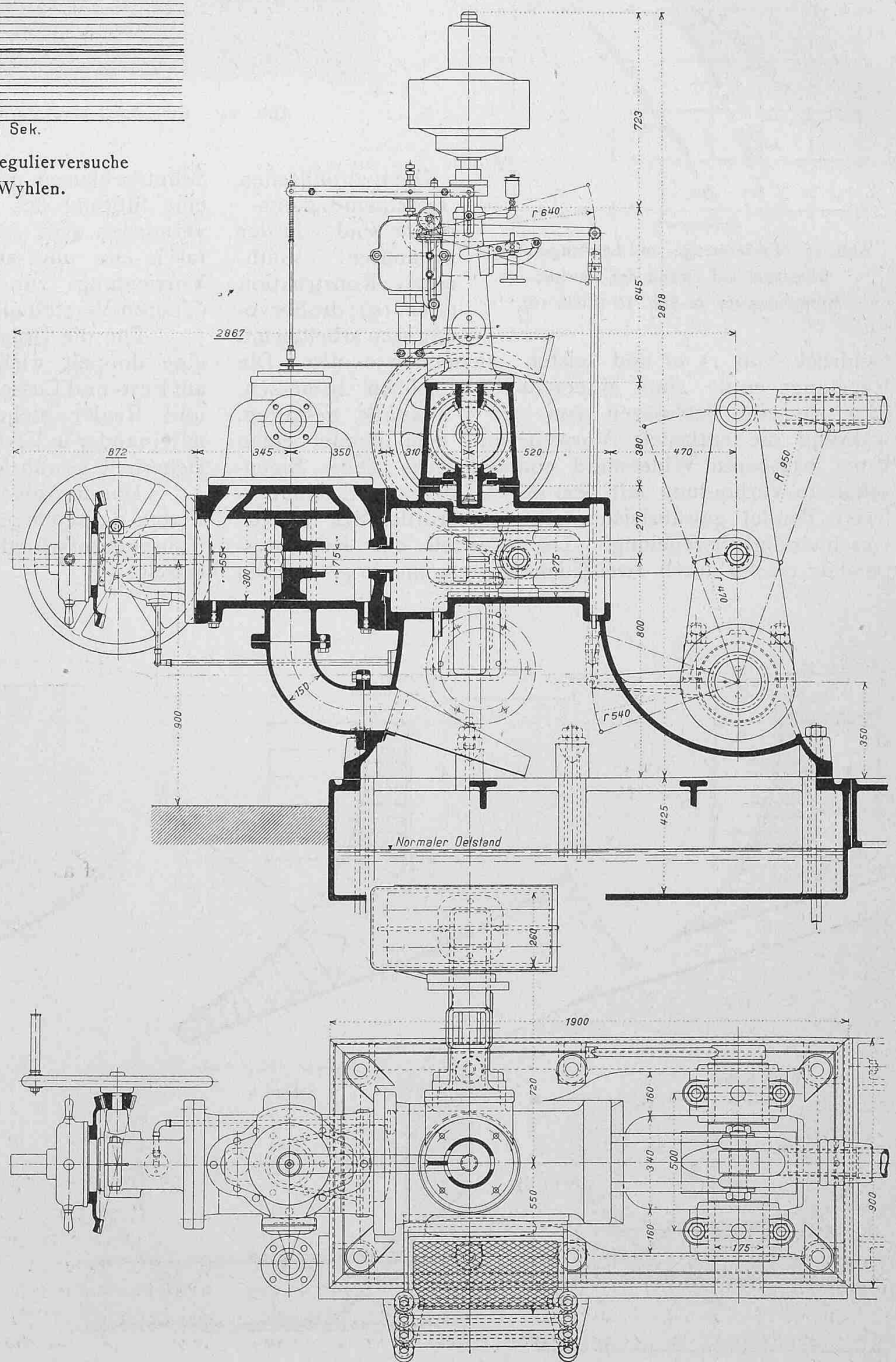
Abb. 19. Turbinen-Regulator Bauart J. M. Voith. — Masstab 1:25.
