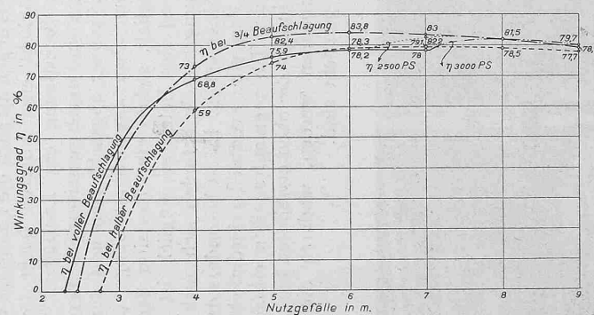
Abb. 16. Wirkungsgrade des in der Versuchsanstalt Hermaringen der Maschinenfabrik J. M. Voith abgebremsten Versuchslaufrades für die Wyhlener Turbinen.
