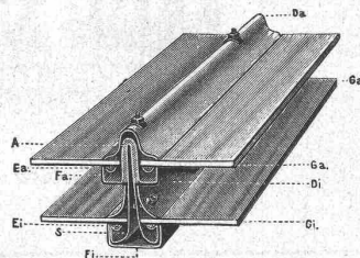
b) Duplexsprosse.
