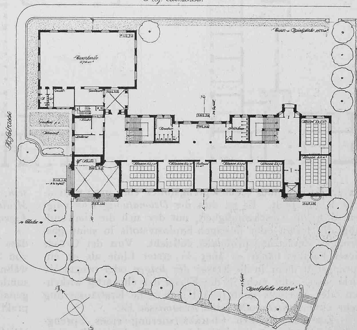
Grundrisse und Schnitt. — Masstab 1:800.
