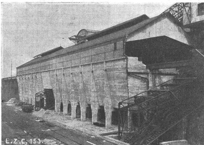
Erztaschenanlage für die Société-Anonyme des Usines de l'Espérance Louvroil près Mabeuge (Nord) Ausgeführt im Jahre 1911. Fassungsvermögen 5600 cbm.
