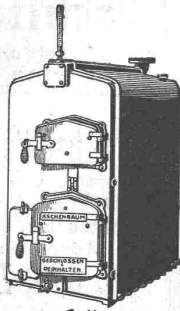
Zollar- Warmwasserkessel.
