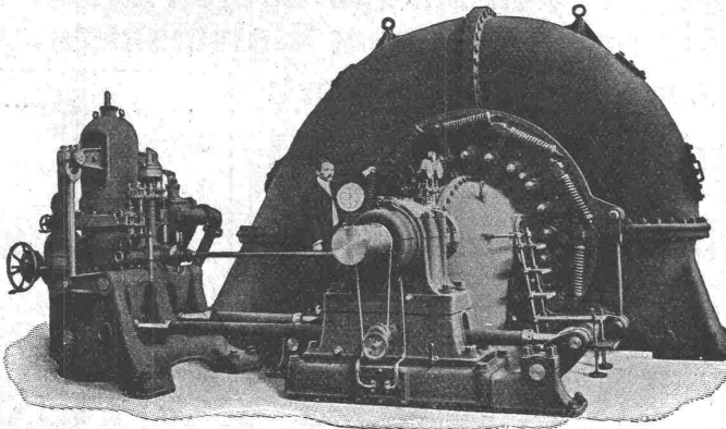
Turbine Francis double de 6200 HP. avec mécanisme de commande des aubes distributrices extérieur à la bêche, orifice compensateur et régulateur à pression d'huile. 50 mètres de chute, 300 tours par la minute.
