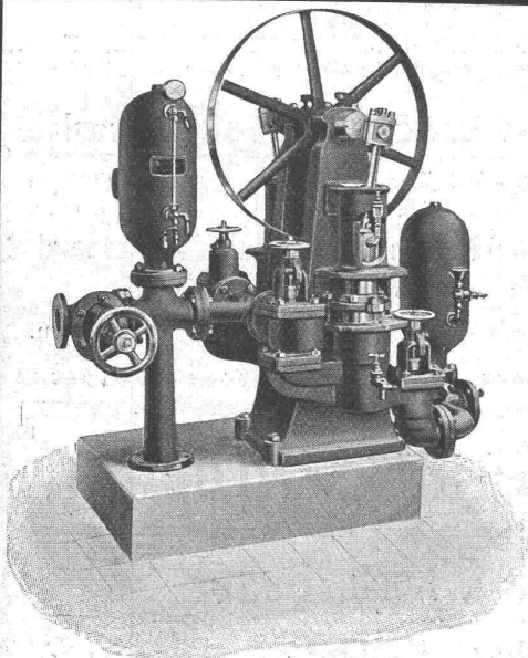
Kolbenpumpen
