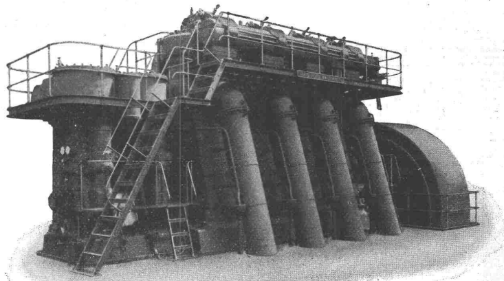
2400 PS-Sulzer-Diesel-Zweitaktmotor.
