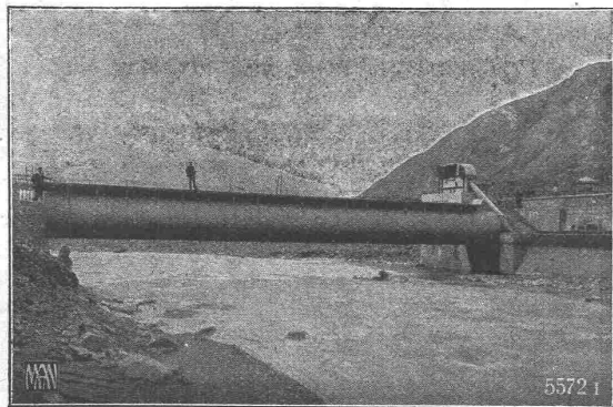
Walzenwehr in der Trisanna bei Landeck in Tirol. I
