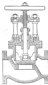
Stahlguss-Ventile mit Patentedichtung.
