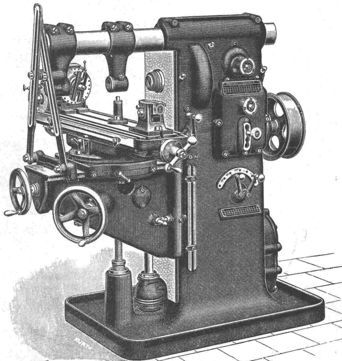
Wanderer-Rapid-Fräsmaschine Nr. 2 mit Einzelscheiben-Antrieb.
