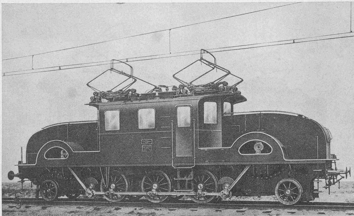
Abb 3. Badische Wiesentalbahn-Schnellzugslokomotive für Einphasenwechselstrom. Von den Siemens-Schuckert-Werken in Verbindung mit J. A. Maffei.
