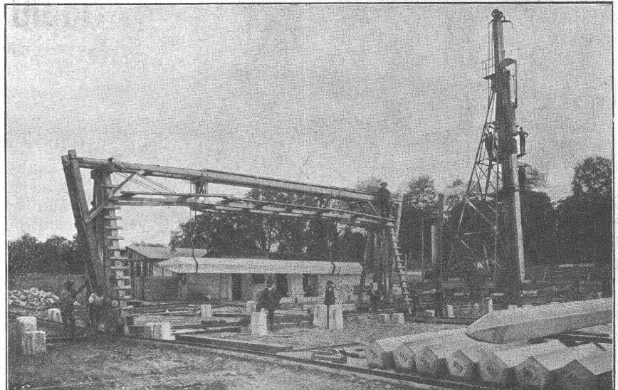
Gründung des Regierungsgebüudes in Düsseldorf mittelst gerammten Eisenbetonpfählen.
