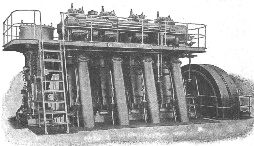
1500 PS Sulzer-Diesel-Zweitaktmotor
