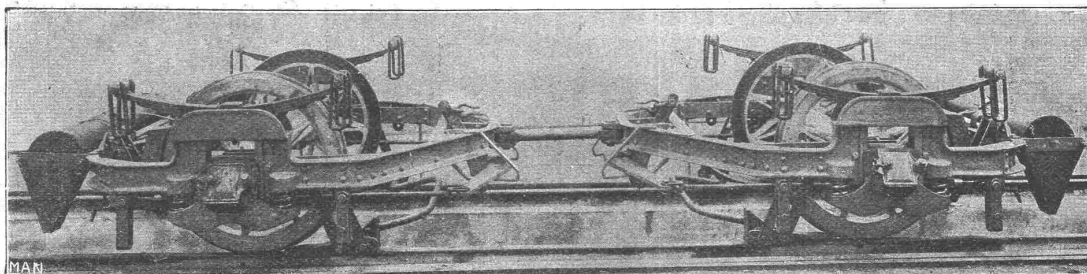
Einachsiges Drehgestell für Motorwagen.
