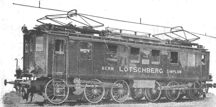
2000 PS Einphasenlokomotive der Lötschbergbahn.
