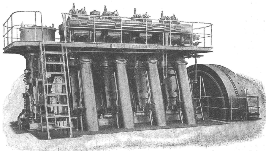
1500 PS Sulzer-Diesel-Zweitaktmotor
