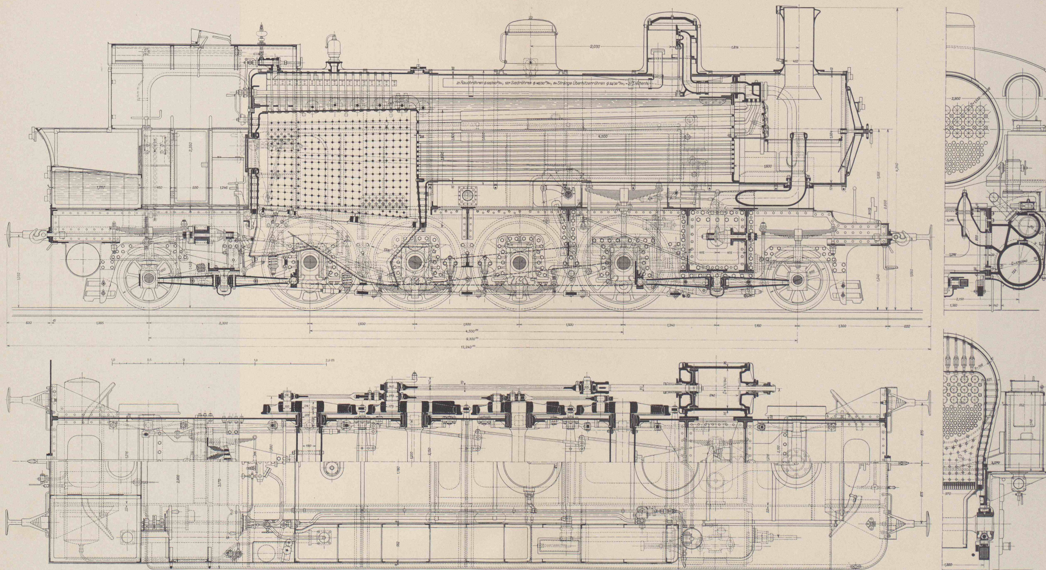
Heissdampf-Tenderlokomotive Serie E c 4/6 der Thunerseebahn, gebaut von der Schweiz. Lokomotiv- und Maschinenfabrik Winterthur
