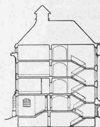
Schnitt. — 1:800.
