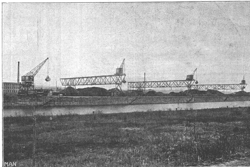
4 elektrisch betriebene Verladebrücken, 72 und 92 m lang, mit Drehkränen, 4000 kg Tragfähigkeit. 2 elektr. betriebene Portal-Drehkrane, 4000 u. 8000 kg Tragfähigkeit. Hafenanlage Offenbach a. M.
