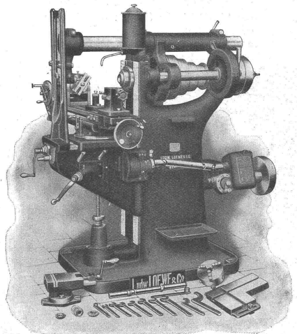
Universal-Fräsmaschine mit Räderkasten Nr. 15, Modell I.
