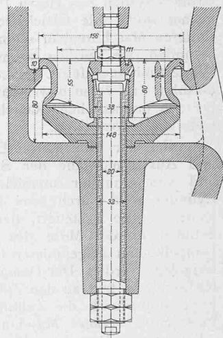
Abb. 3. Querschnitt durch Zylindermitte und Auslassöffnungen. Masstab 1 : 20.
