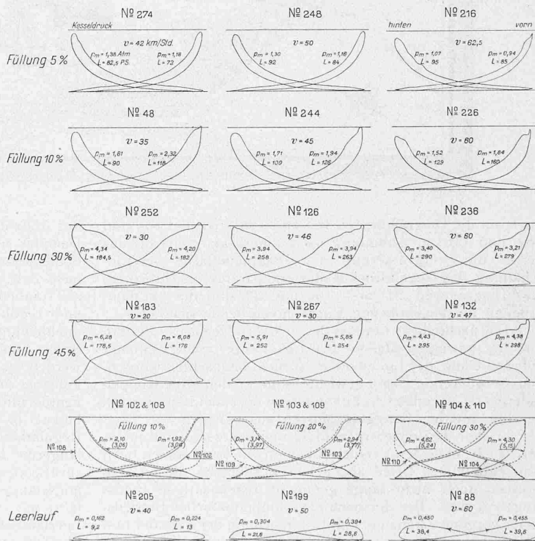
Abb. 10. Indikatordiagramme der C 4/6 Lokomotive, Bauart Stumpf.
