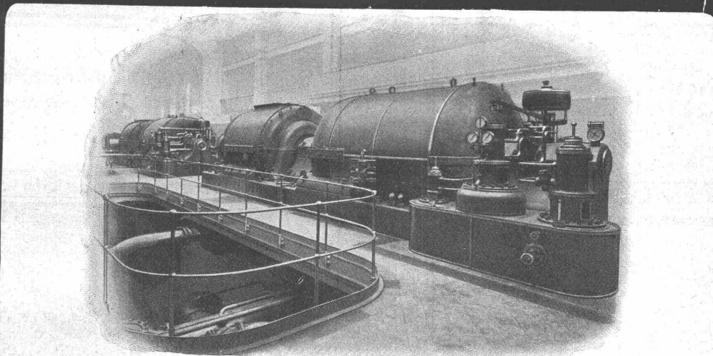
10 000 PS Oerlikon-Turbogeneratoren im Elektrizitätswerk Stockholm
