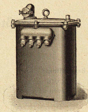
Fig. 3. Drehstromtransformator mit Selbstkühlung, Modell KO.
