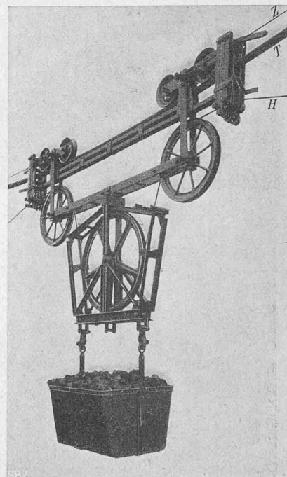
Abb. 14. Laufwagen mit den Seilreitern.
