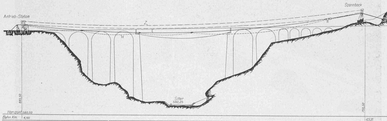
Abb. 9. Längenprofil der Kabelbahn I. — Masstab 1:2500. — Legende: ——— Tragseil, - - - - Zugseil, — — — Hubseil.
