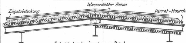
Schnitt durch ein ebenes Dach
