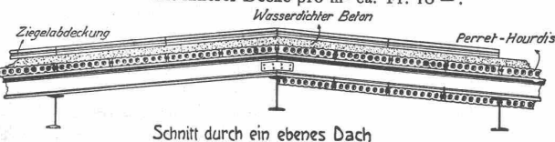
Schnitt durch ein ebenes Dach
