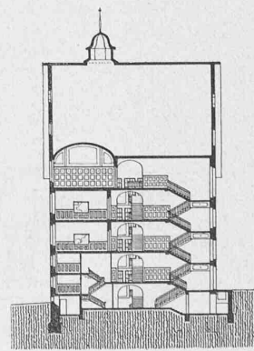
Schnitt. — Masstab 1:800.
