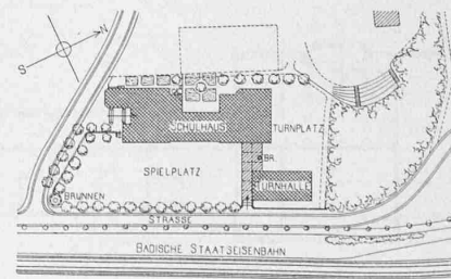
Lageplan. — Masstab 1:3000.
