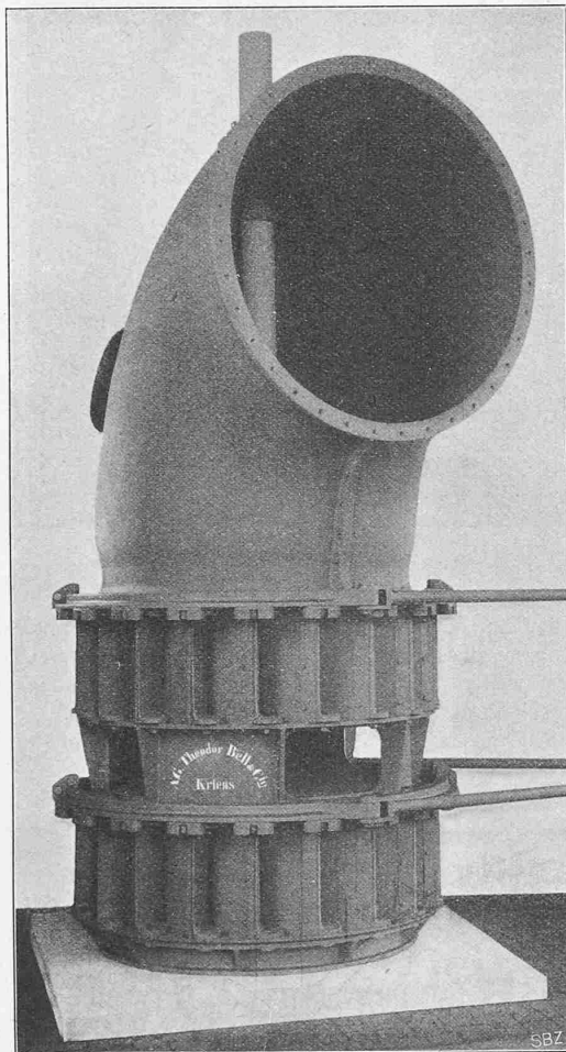
Abb. 15. Doppel-Francis-turbine für Hoch- und Niederwasser gebaut vo Th. Bell & Co. in Kriens.
