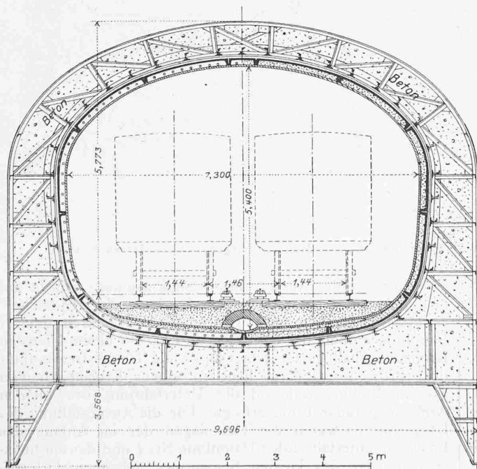
Abb. 2. Querschnitt der Caisson-Tunnelstrecke. — 1 : 100.
