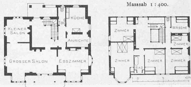
Abb. 1 u. 2. Grundrisse vom Erdgeschoss und I. Stock der Villa Gardy.
