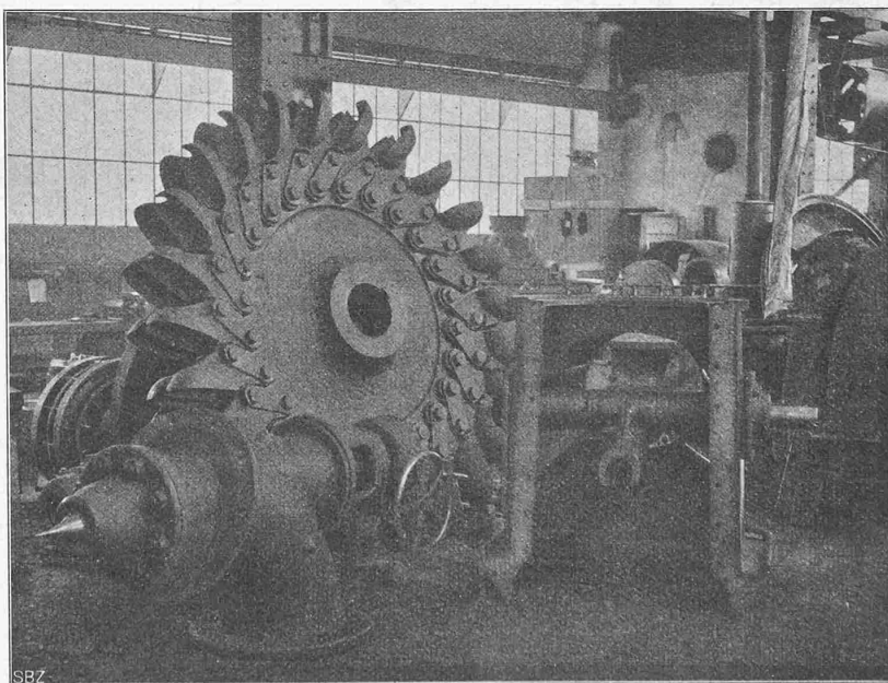
Abb. 24. Rad, Nadeldüse und Strahlablenker der 5500 PS-Turbine.
