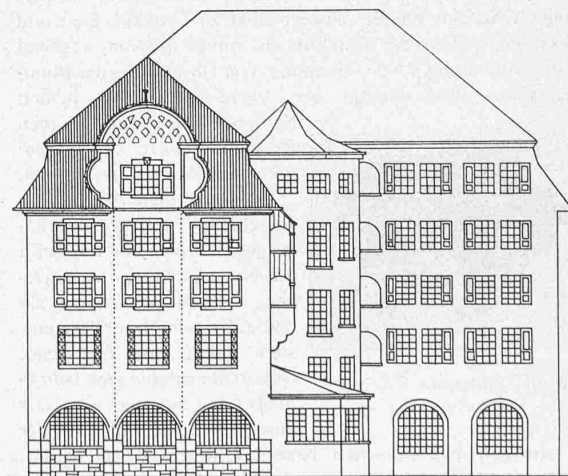
Seiten- und Hofansicht. — Masstab 1 : 400.
