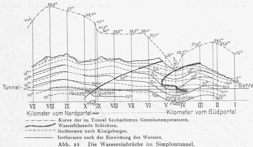
Abb. 22 Die Wassereinbrüche im Simplontunnel.
