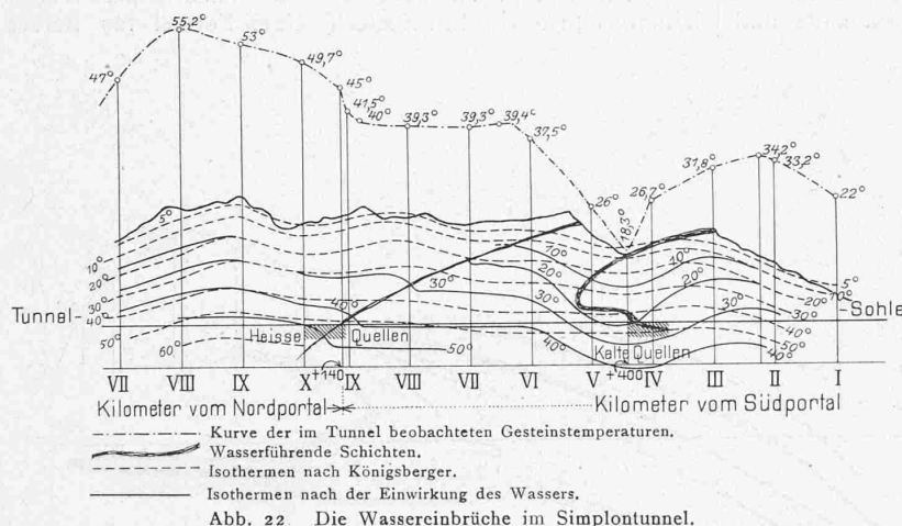
Abb. 22 Die Wassereinträge im Simplontunnel. Isothermen im Gestein konstruiert nach den beobachteten Gesteinstemperaturen im Tunnel.
