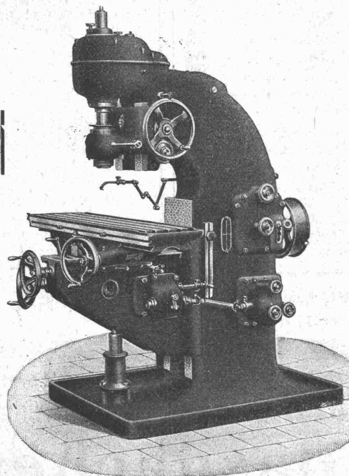
Vertikal-Fräsmaschine Nr. 3.
