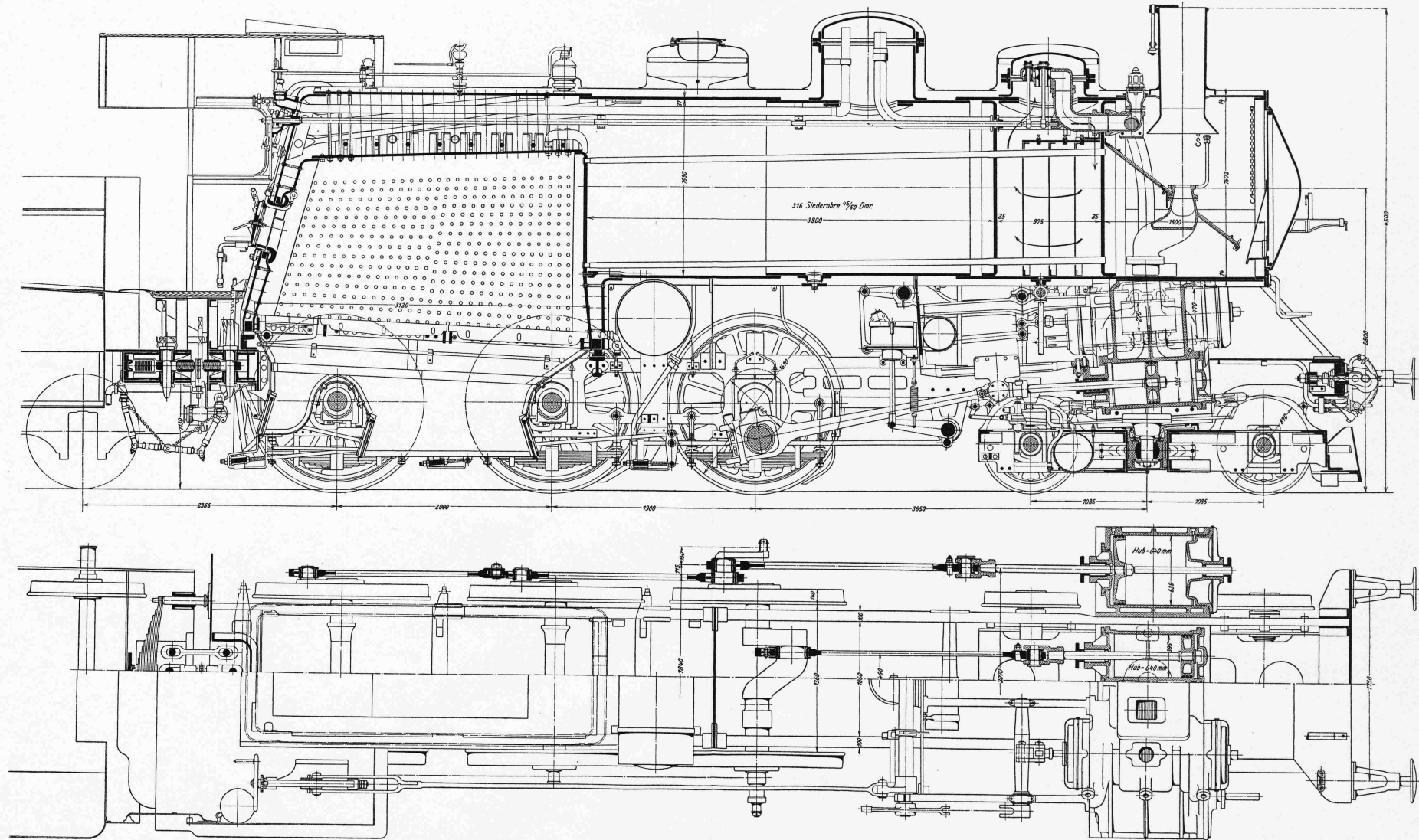
Die neue Vierzylinder-Verbund-Lokomotive mit drei gekuppelten Achsen der Gotthardbahn — Serie A 3 / 5 .
