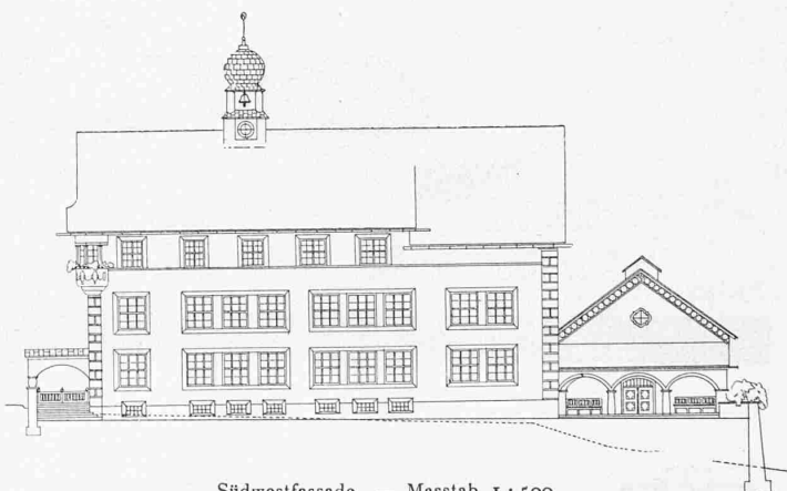
Südwestfassade. — Masstab 1 : 500.
