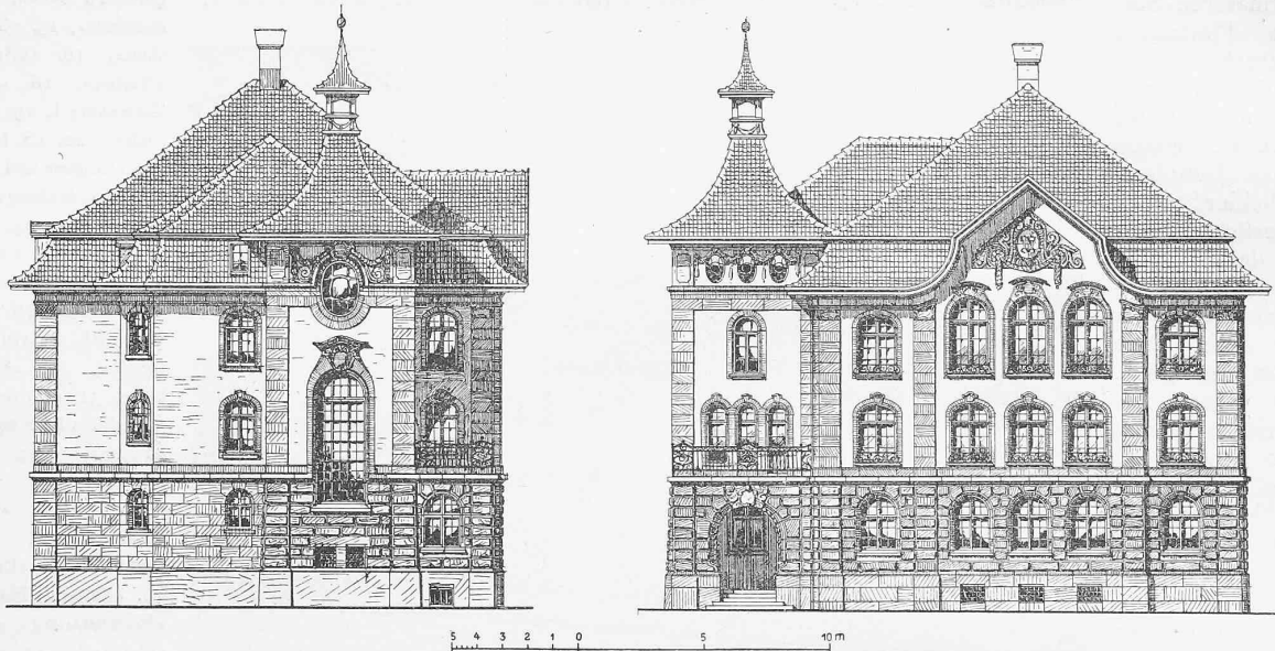
Geometrische Ansicht der Ostfassade sowie der nördlichen Hauptfront. — Masstab 1 : 300.
