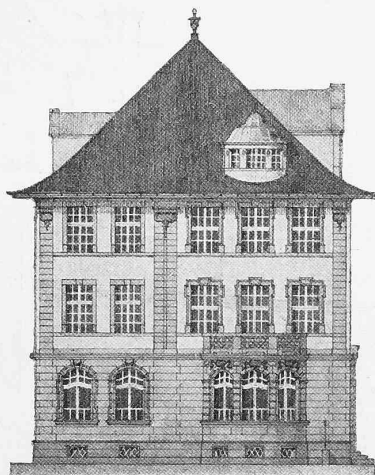
Gemetrische Ansicht der Ostfassade sowie der nördlichen Hauptfront. — Masstab 1:300.
