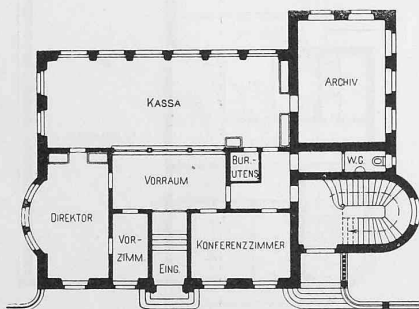
Grundrisse vom Erdgeschoss, vom ersten Obergeschoss und vom Dachstock. — Masstab 1:400.
