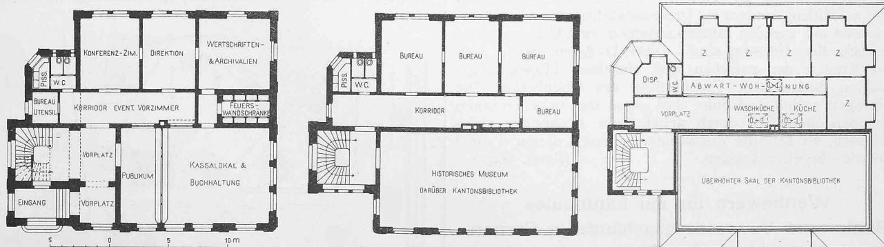
Grundrisse vom Erdgeschoss, vom ersten Obergeschoss und vom Dachstock. — Masstab 1:400.
